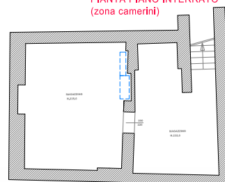
PIANTA PIANO INTERRATO (zona camerini)
