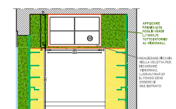
SEZIONE C-C'
